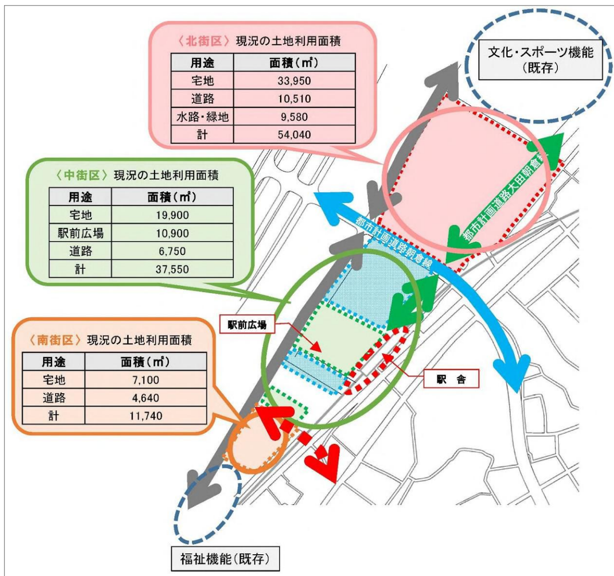
朝倉駅周辺整備事業の街区分図
